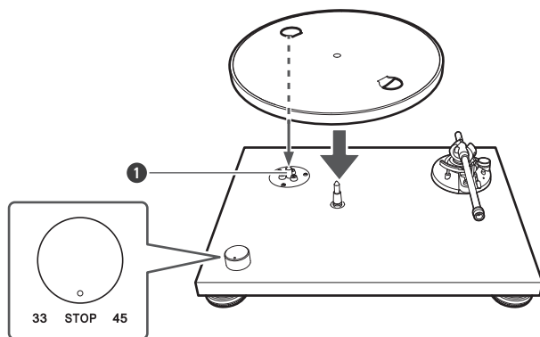
❶ 电机滑轮（黄铜色）
