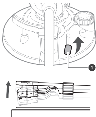
① 唱臂升降控制杆
