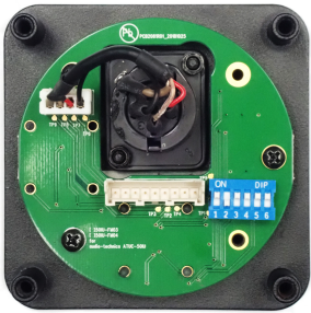
后视图
